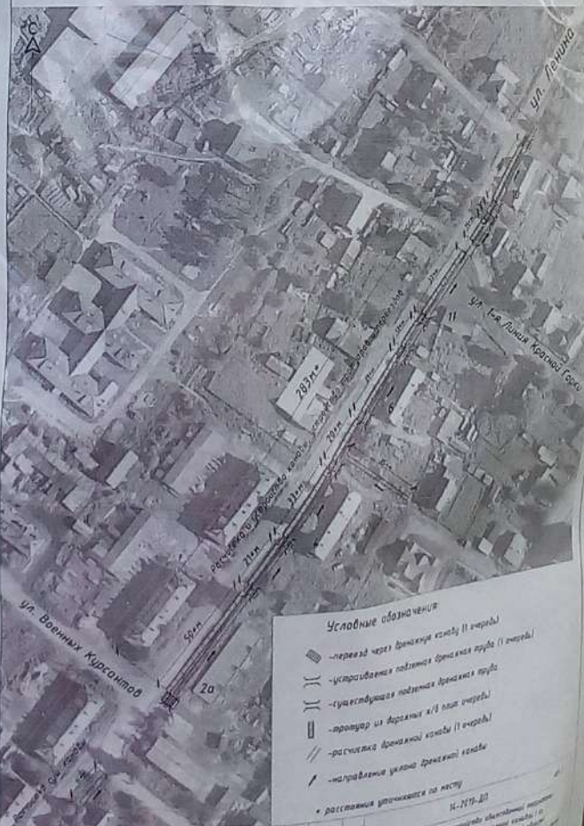
Схема расположения тротуаров с дренажной канавой по ул.Ленина М1:1000
